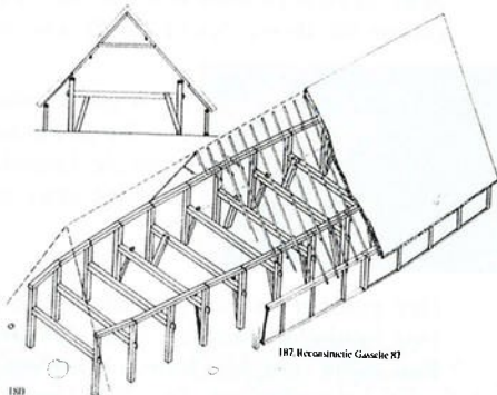
Reconstructie huistype Gasselte
