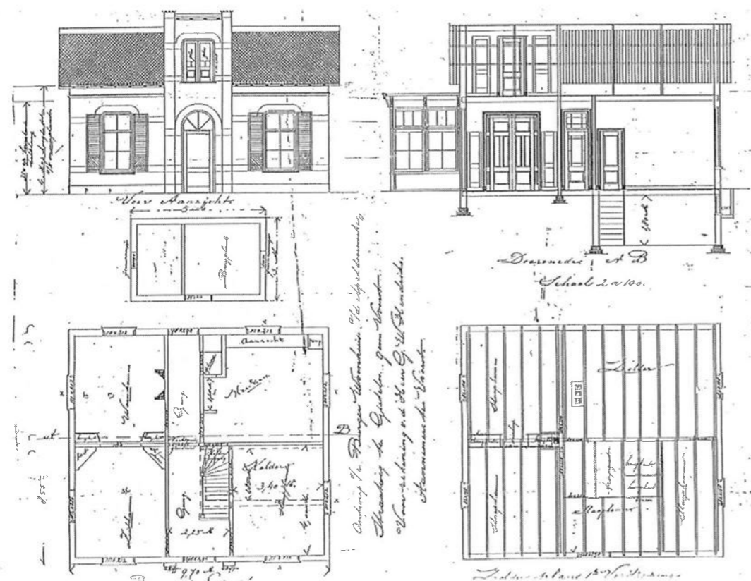
Bouwtekening Villa Johanna (Rijksstraatweg 18) ook wel genoemd Mon Repos.
